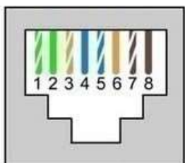
T568A
