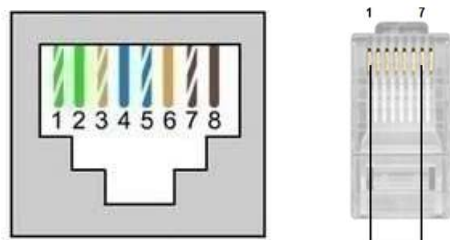
T568A
